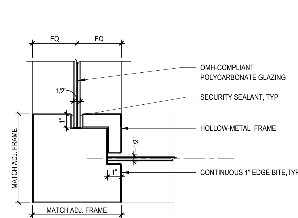
D2 HM WINDOW CORNER - BH 3" = 1'-0"
