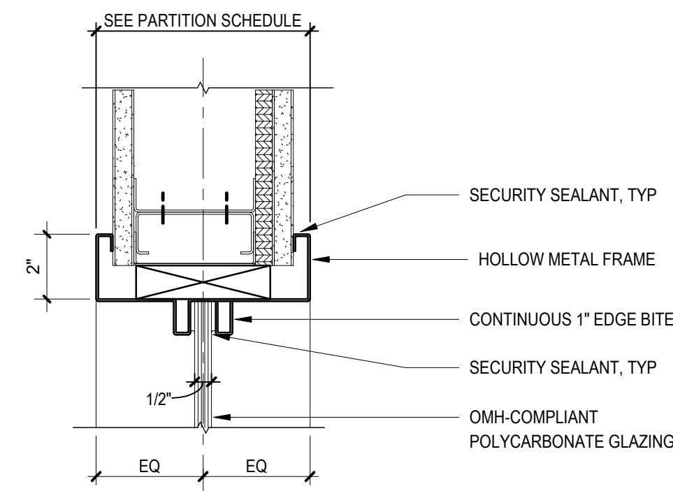
D1 HM WINDOW HEAD - BH 3" = 1'-0"
